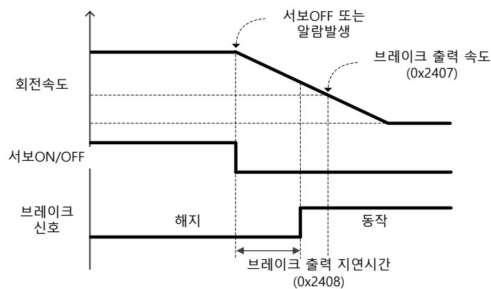
브레이크 출력 지연시간(0x2408)에 의한 신호출력 시 타이밍도
