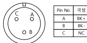
Plug : MS3102A14-7P
