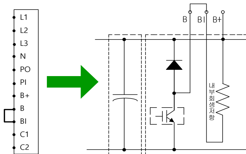
내부 회생 저항 사용 시 배선 방법
