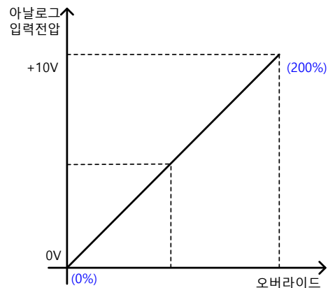
0x221E : 2 일때
