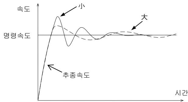
(4) 속도 명령 필터 및 속도 피드백 필터 설정
