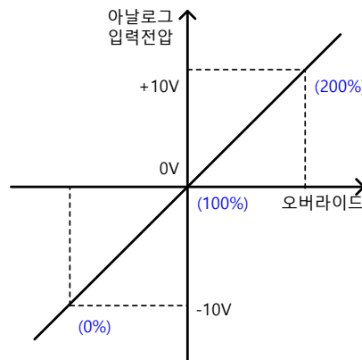
0x221E : 1 일때
