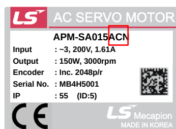
Incremental(증분형)
